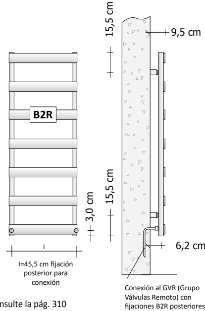
VERSIÓN HIDRÁULICA ESTÁNDAR (Fijaciones B2R)
