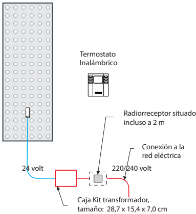
Conexión mediante termostato de Pared Inalámbrico (ZRF007)
