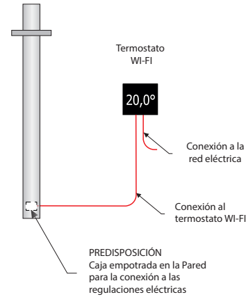
Conexión mediante termostato «ZRF» de Pared WI-FI (ZRF081 - ZRF082)
