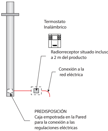
Conexión mediante termostato de Pared Inalámbrico (ZRF007)
