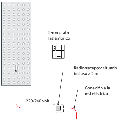
Conexión mediante termostato de Pared Inalámbrico (ZRF007)
