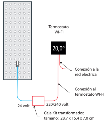
Conexión mediante termostato «ZRF» de Pared WI-FI (ZRF081 - ZRF082)
