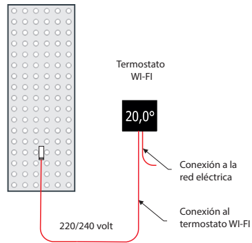
Conexión mediante termostato «ZRF» de Pared WI-FI (ZRF081 - ZRF082)
