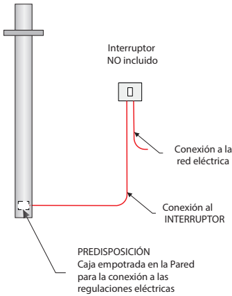
Conexión directa al interruptor (no incluido) o a la instalación domótica doméstica
